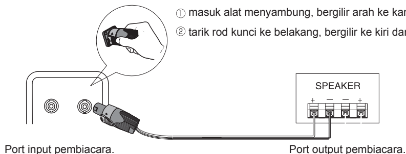
Gambar sirkuit skematis pembicara.
