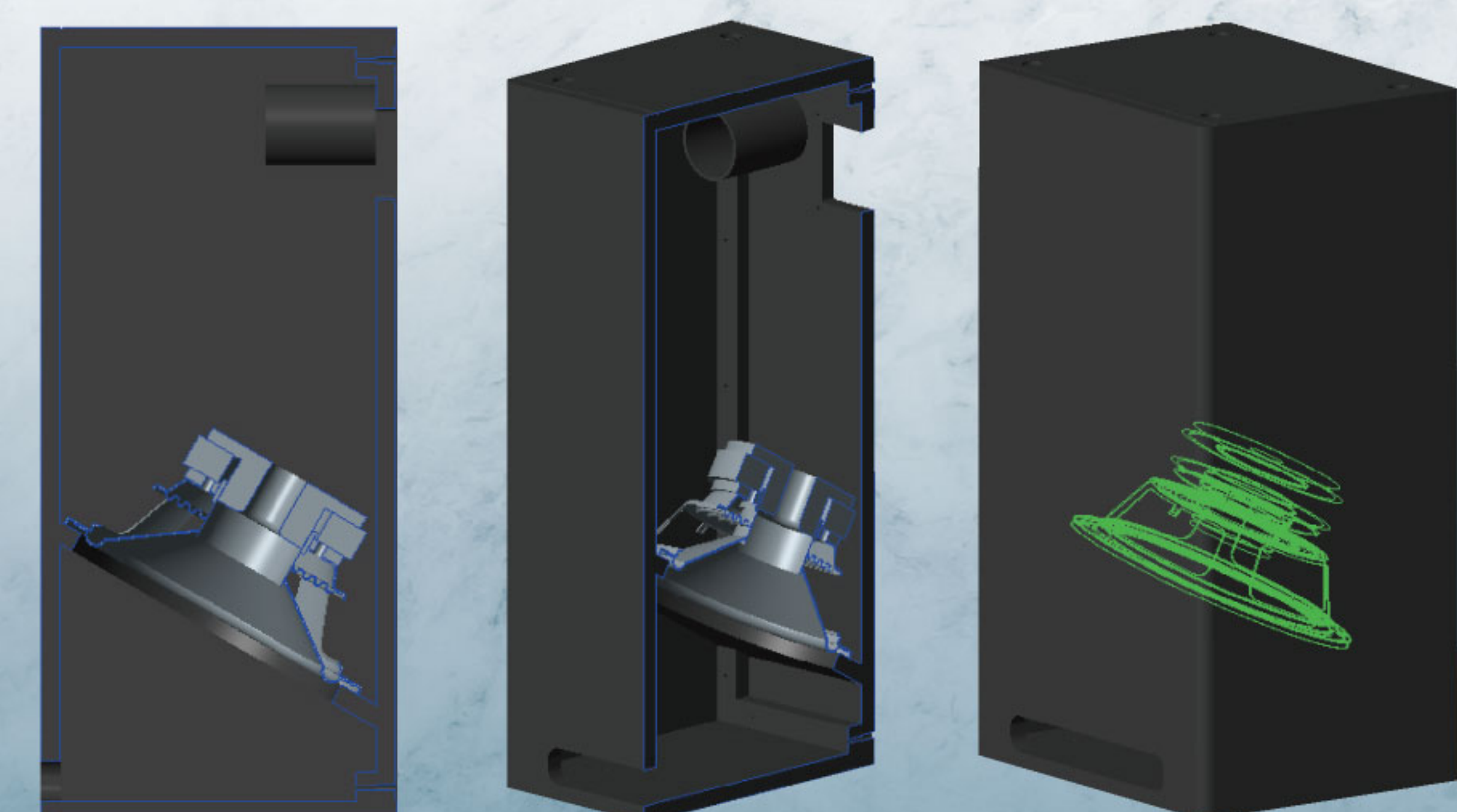
■ 低音炮构造 双音圈系统
